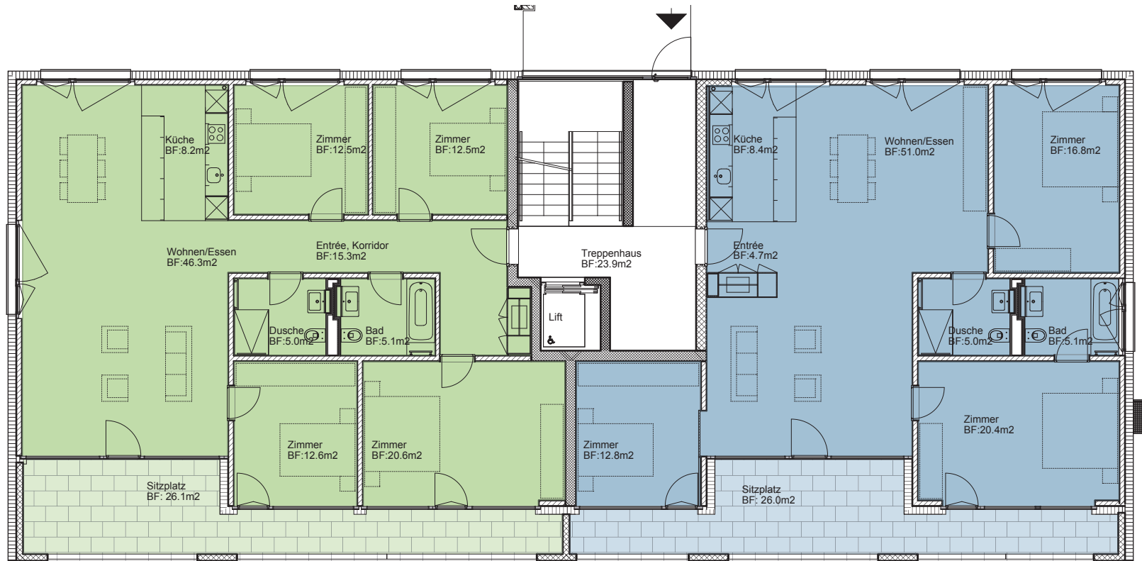
WOHNUNG NR. A11 5.5-ZIMMERWOHNUNG WOHNFLÄCHE 138.1m 2 SITZPLATZ 26.1m 2
