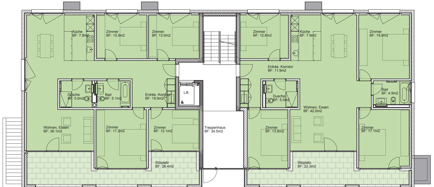
WOHNUNG NR. C11 5.5-ZIMMERWOHNUNG WOHNFLÄCHE 128.3m 2 SITZPLATZ 28.4m 2
